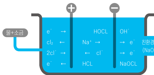
살균수 생성 원리
